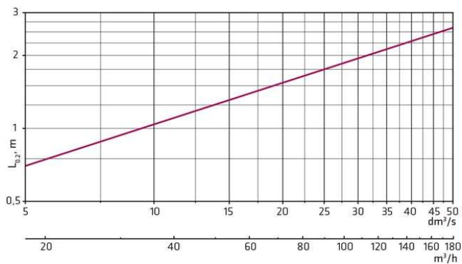
ECO-C – dosah proudu (změna teploty přívodního vzduchu dosah neovlivňuje)
