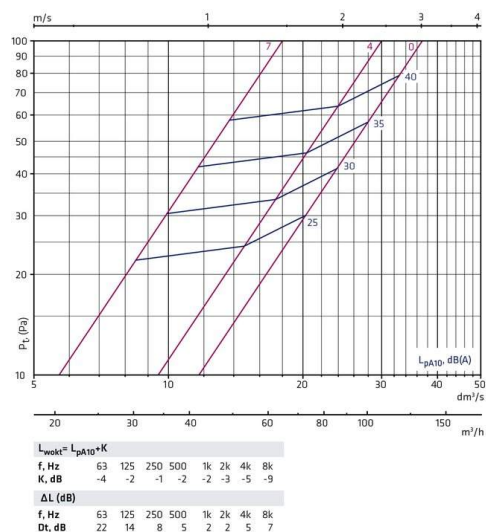
ECO-C – tlaková ztráta a hladina akustického tlaku
