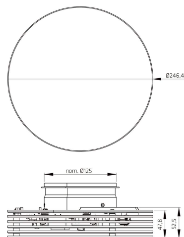
ECO-C – hlavní rozměry
