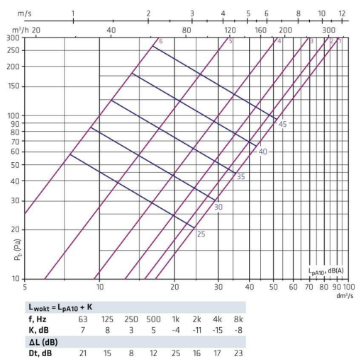
HALOI-160 + FLO-100-160 · odvod
