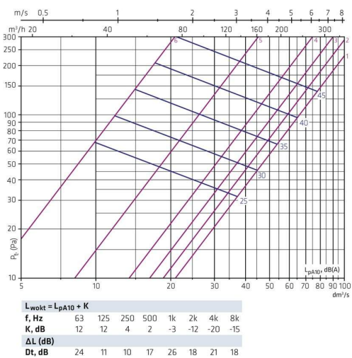
HALOI-125 + FLO-125-125 · odvod
