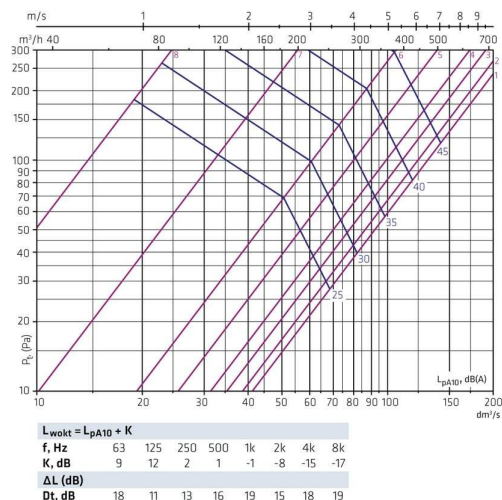
HALO-200 + FLO-160-200 · přívod
