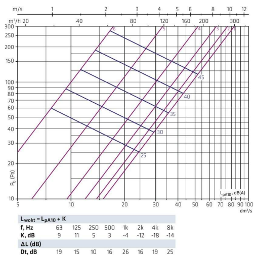
HALOI-125 + FLO-100-125 · odvod
