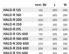
HALO-R – hlavní rozměry
