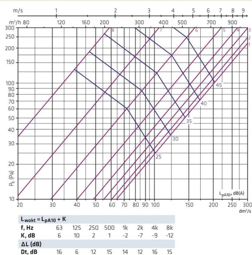
HALO-315 + FLO-200-315 · přívod
