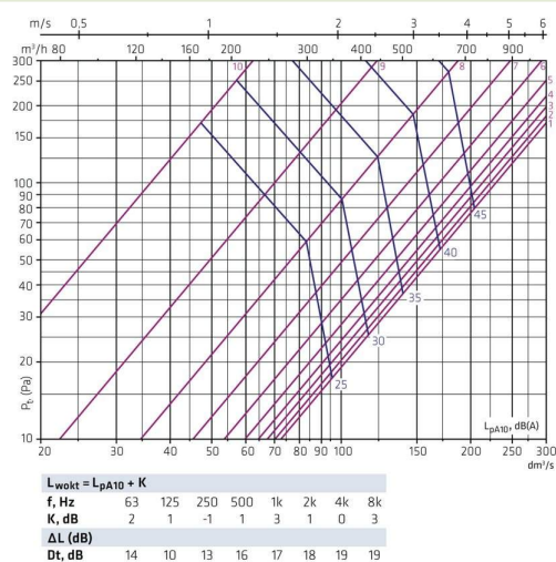
HALO-250 + FLO-250-250 · přívod
