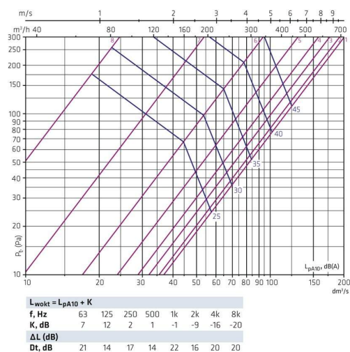
HALO-160 + FLO-160-160 · přívod
