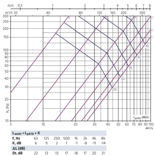
HALO-160 + FLO-125-160 · přívod
