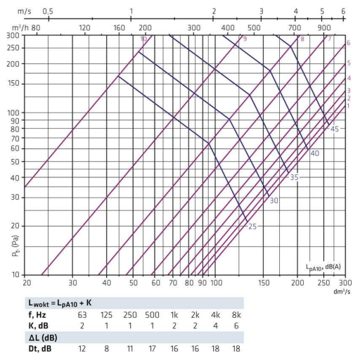
HALO-315 + FLO-250-315 · přívod
