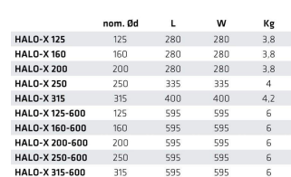
HALO-X – hlavní rozměry
