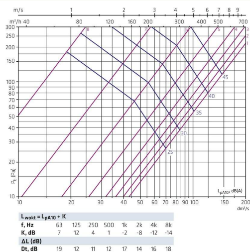
HALO-250 + FLO-160-250 · přívod
