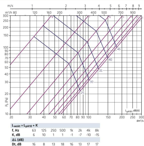
HALO-250 + FLO-200-250 · přívod
