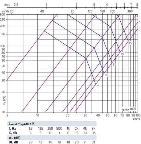
HALO-125 + FLO-125-125 · přívod
