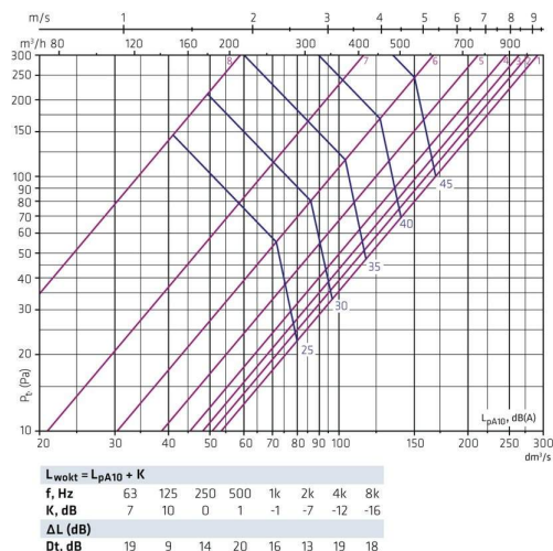
HALO-200 + FLO-200-200 · přívod
