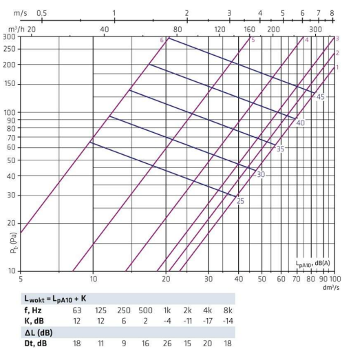
HALOI-160 + FLO-125-160 · odvod
