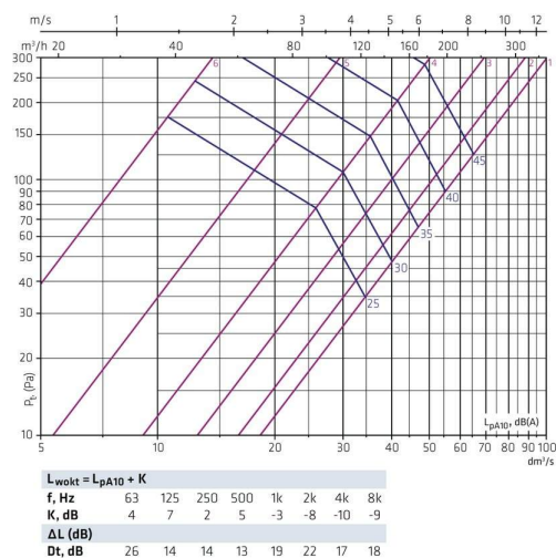
HALO-160 + FLO-100-160 · přívod
