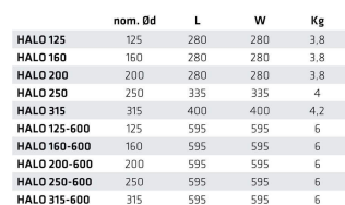
HALO – hlavní rozměry
