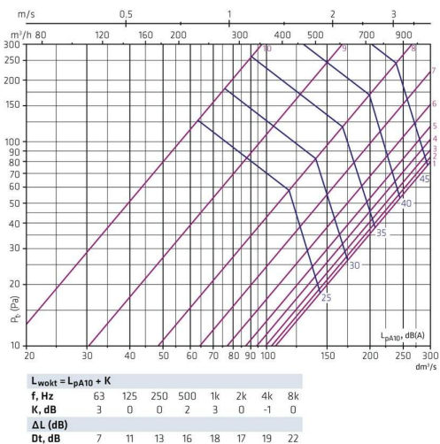
HALO-315 + FLO-315-315 · přívod
