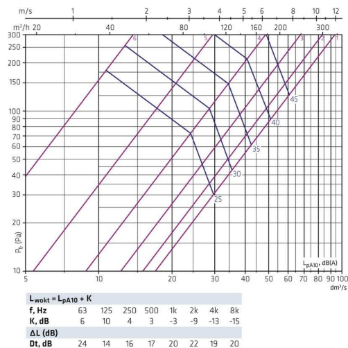
HALO-125 + FLO-100-125 · přívod
