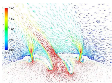
1 · Přívodní vzduch se účinně mísí s okolním – vyrovnává teploty a snižuje rychlosti v pobytové zóně
