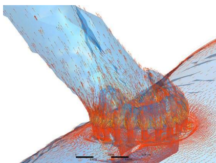
2 · Konstrukce brání proudů narážet na povrch – nečistoty ze sekundárního vzduchu neulpívají
