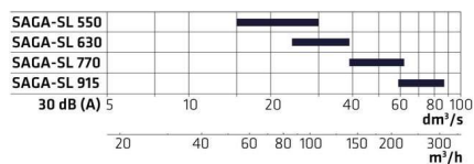
Quick guide – přívod
