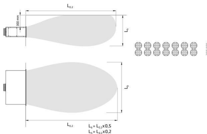
Čelní dlouhé a úzké vyústění
