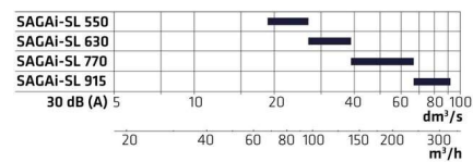
Quick guide – odvod
