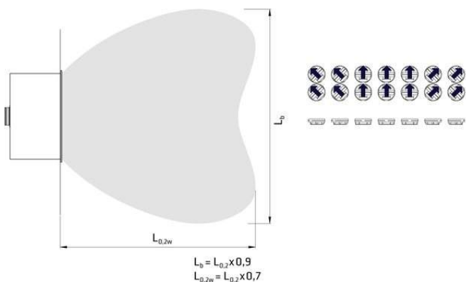
Čelní krátké vyústění
