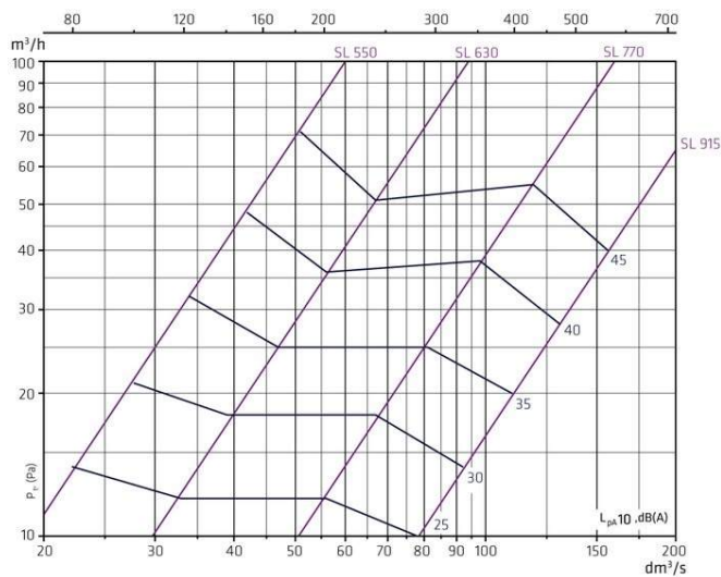
SAGA-SL – dimenzování · odvod
