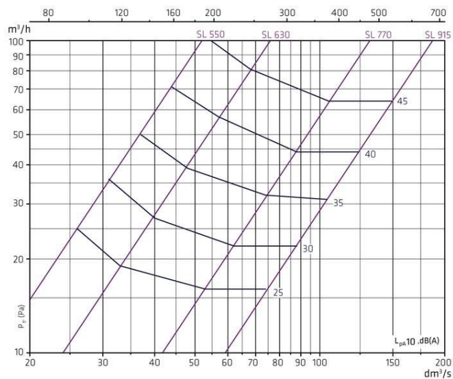
SAGA-SL – dimenzování · přívod
