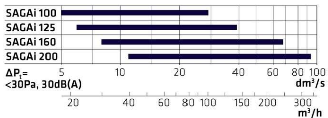
Quick guide – odvod (SAGAi)
