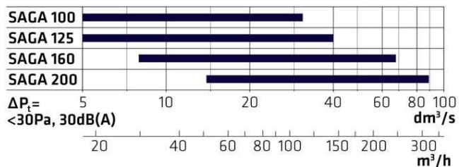
Quick guide – přívod (SAGA)
