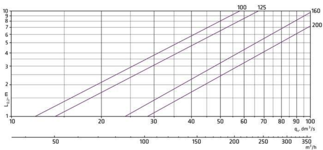
Dosah proudu v závislosti na průtoku
